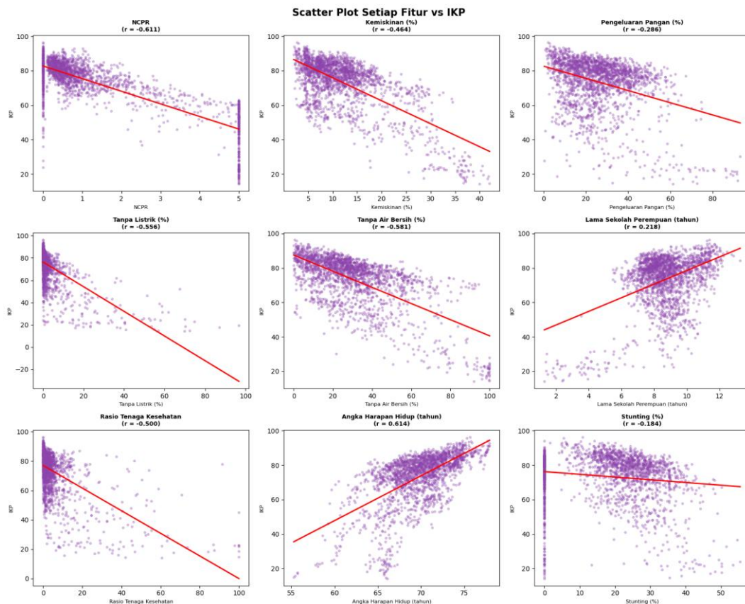
Gambar 4. Scatter Plot Setiap Fitur terhadap IKP dengan Garis Tren dan Korelasi Spearman
